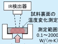
熱伝導率測定(フラッシュ法)
